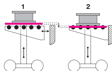
Versione del carrello di cambio stampi senza ponte con stazione di aggancio di sicurezza e tavola a sfere
