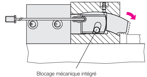
Blocage mécanique intégré
