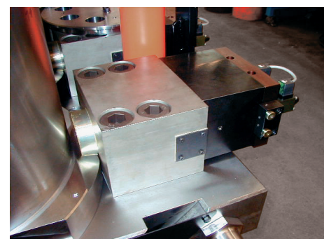
Elementi di bloccaggio a cuneo su una forgia
