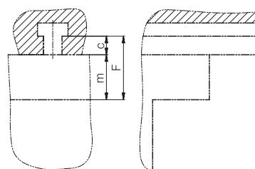
Dimension de serrage F = c + m
