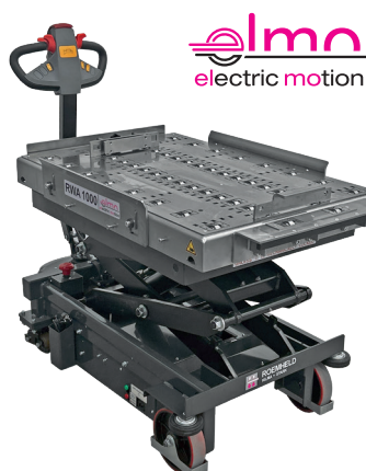
Ejecución RWA1000 elmo con mesa de rodillos
